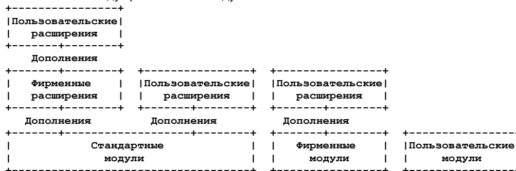
Рисунок 2. Варианты происхождения модулей YANG.
