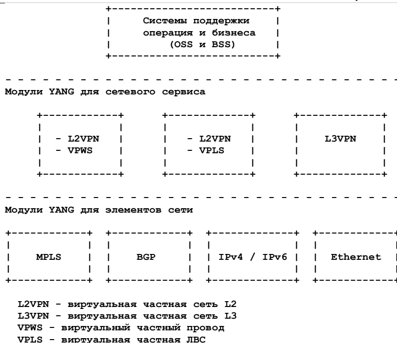
Рисунок 1. Абстрактные уровни модулей YANG.
