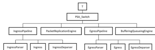
Рисунок 3. Дерево минимального экземпляра PSA.
