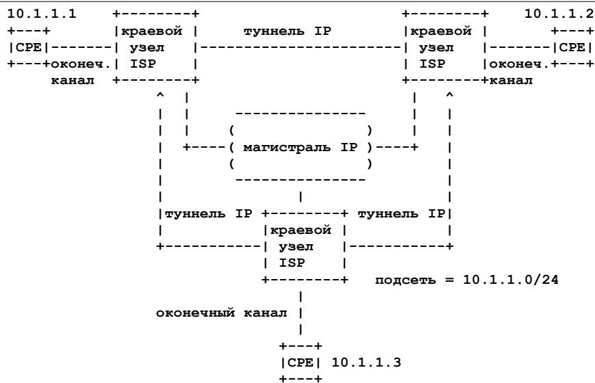
Рисунок 7.1. Пример VPLS.
