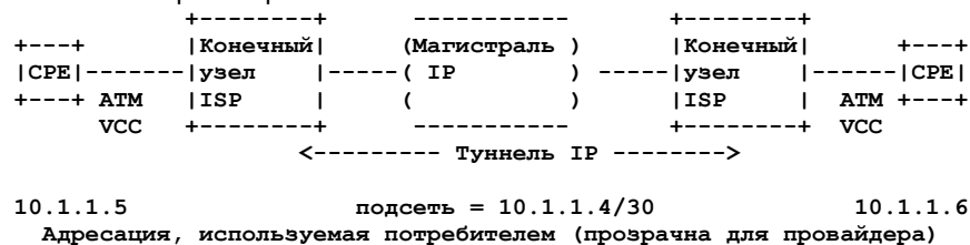
Рисунок 4.1. Пример VLL.
