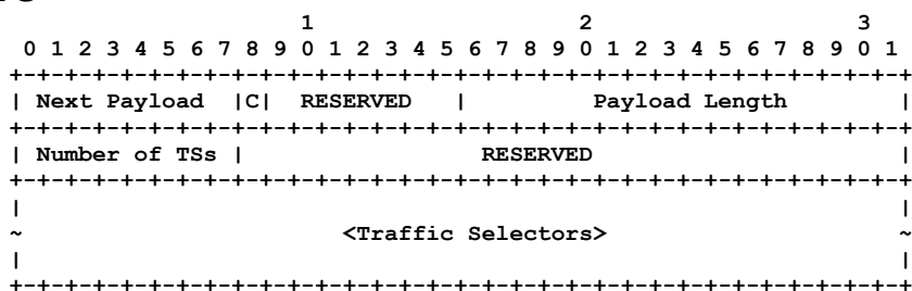
Рисунок 19. Формат элемента TS.
