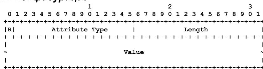
Рисунок 23. Формат атрибута Configuration.
