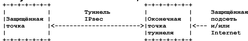
Рисунок 3. Туннель между конечной точкой и защитным шлюзом.
