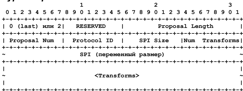
Рисунок 7. Субструктура Proposal.
