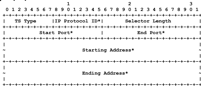
Рисунок 20. Селектор трафика.
