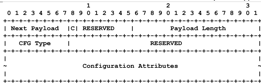
Рисунок 22. Формат элемента Configuration.
