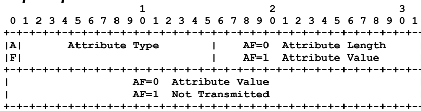
Рисунок 9. Атрибуты преобразования.
