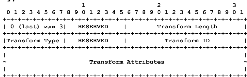
Рисунок 8. Субструктура Transform.
