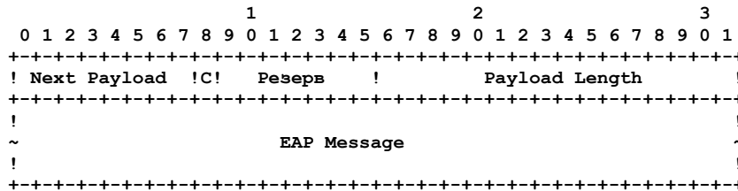
Рисунок 24. Формат EAP.
