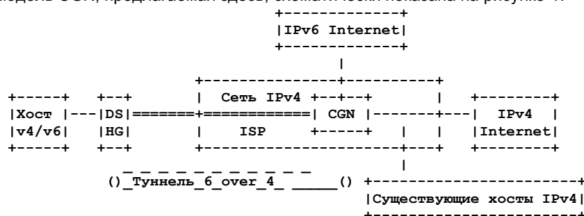
Рисунок 1. Инкрементная модель CGN для сети IPv4 Internet-провайдера DS HG - домашний шлюз с двумя протоколами (CPE - оборудование на стороне пользователя).
