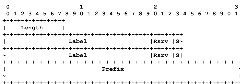
Рисунок 3. NLRI с последовательностью меток.
