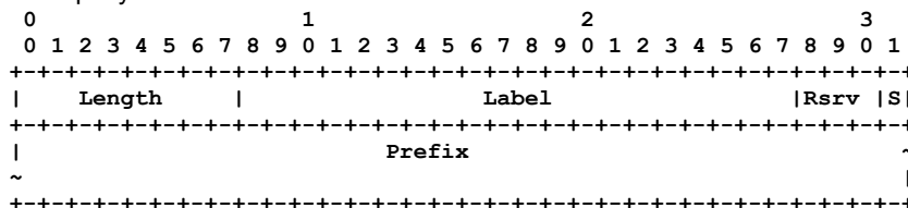
Рисунок 2. NLRI с одной меткой.
