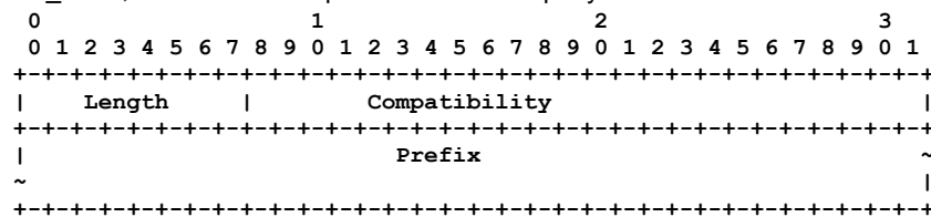
Рисунок 4. NLRI для отзыва.
