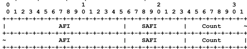
Рисунок 1. Формат Multiple Labels Capability.
