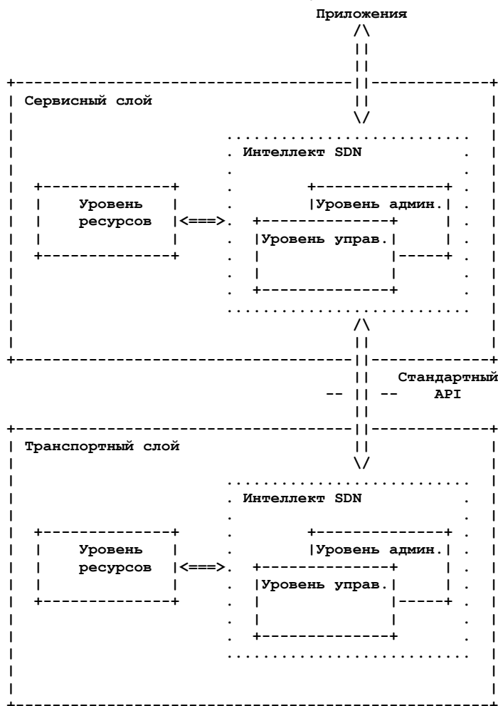
Рисунок 1. Архитектура CLAS.
